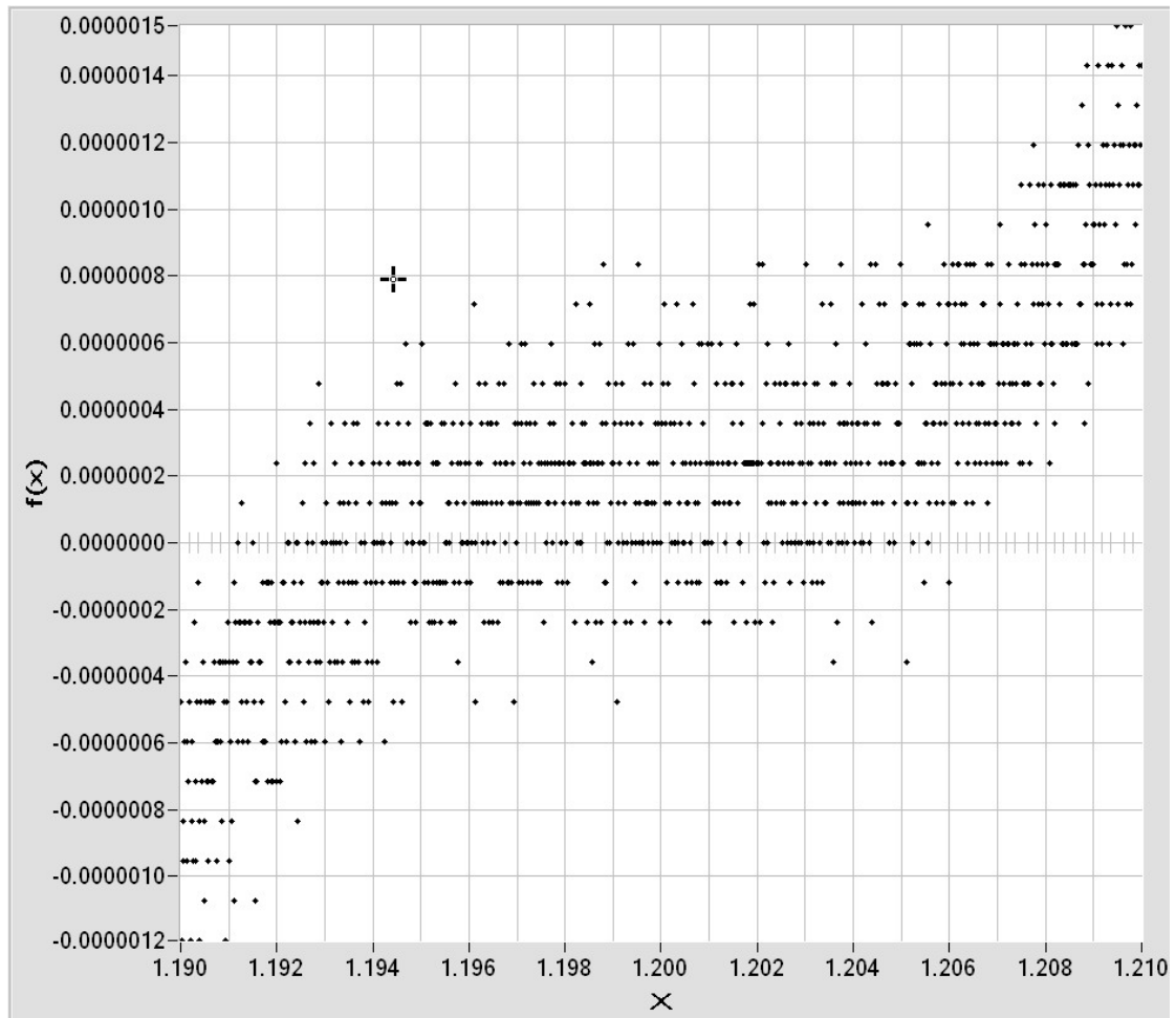
Figura 1 - Zgomot numeric
